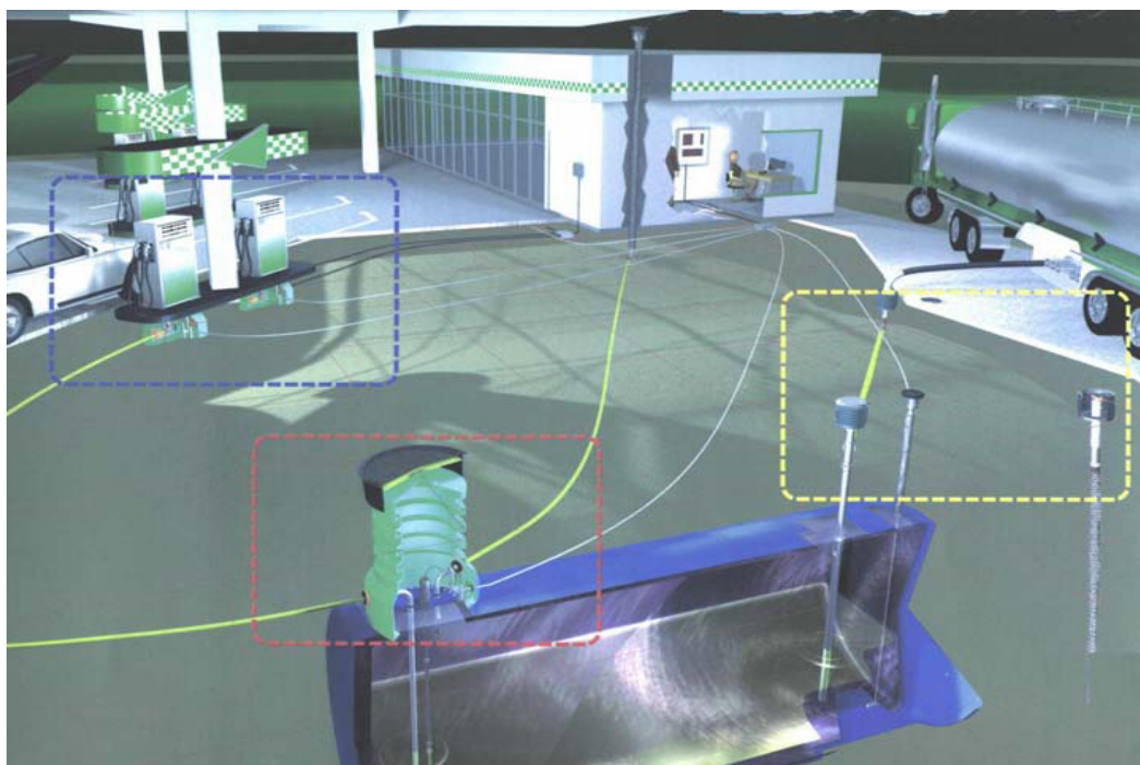
Figura 01 – Esquema típico de um Posto Revendedor de Combustível
