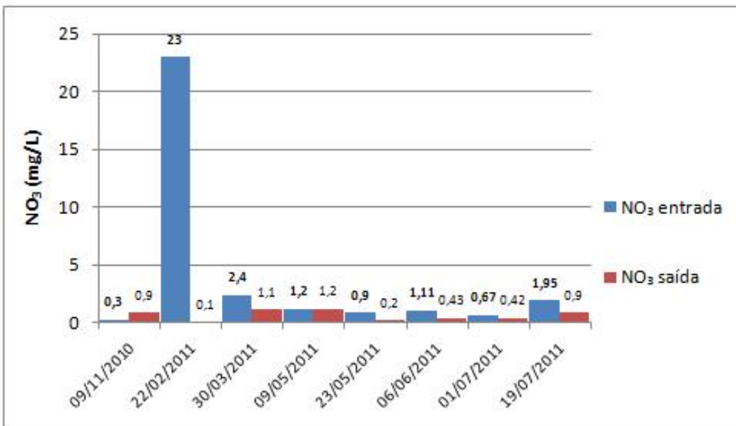
Figura 6 - Variação dos valores de entrada e saída do wetland durante o período avaliado
