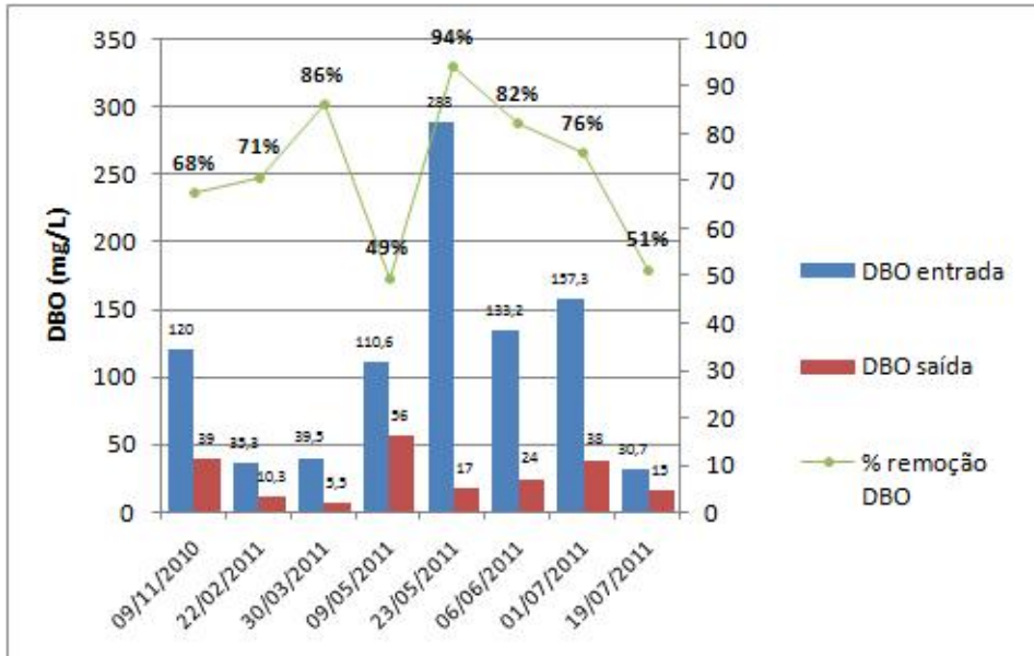
Figura 4 - Valores absolutos de entrada e saída e eficiência média de remoção da DBO
