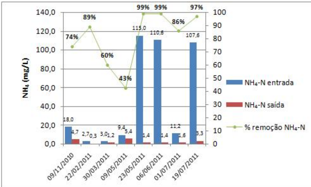
Figura 5 - Variação dos valores de Nitrogênio amoniacal na entrada e saída do sistema por zona de raízes durante o período de avaliação
