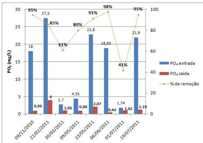
Figura 7 - Variação dos valores do fósforo, entrada e saída dos sistemas por zona de raízes no período avaliado
