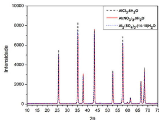
Figura 3 – Difratoformas de Raios X dos resíduos de \text{AlCl}_3 \cdot 6\text{H}_2\text{O} , \text{Al}(\text{NO}_3)_3 \cdot 9\text{H}_2\text{O} e \text{Al}_2(\text{SO}_4)_3 \cdot (14-18)\text{H}_2\text{O} obtidos a 1200 °C
